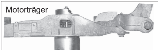
Ausbau
